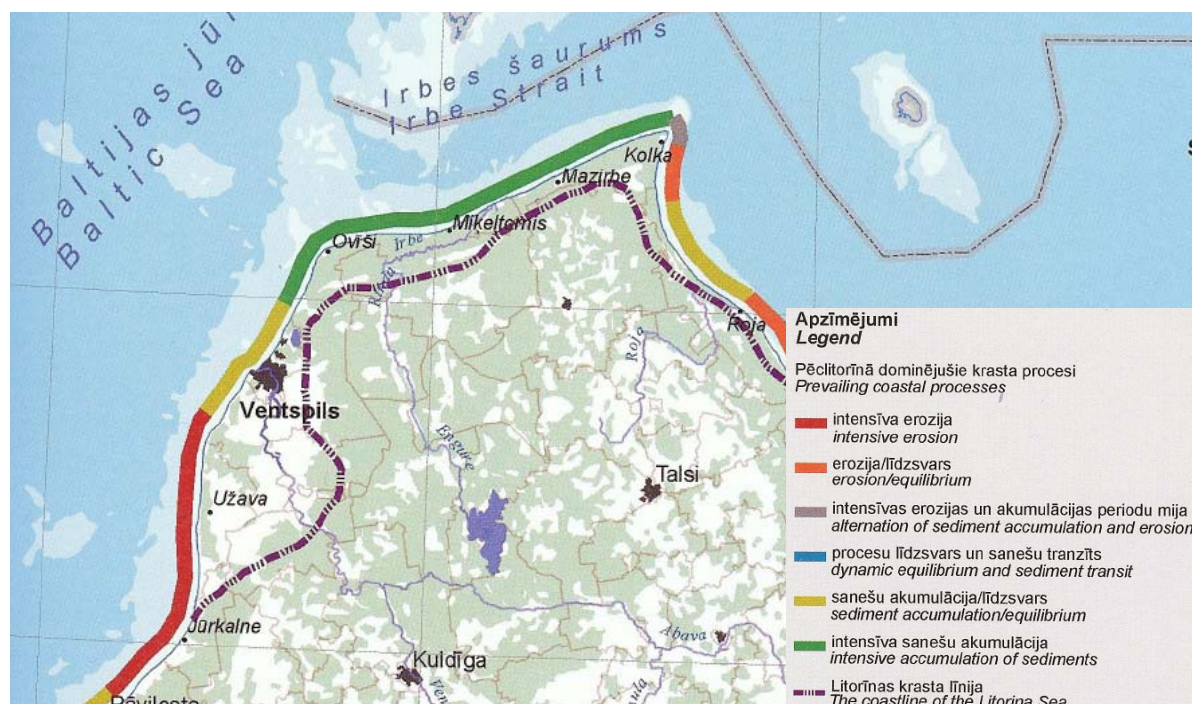
8. attēls. Krasta procesi pēc Litorīnas jūras regresijas. Avots: Baltijas jūras Latvijas krasta procesi. Atlants. Guntis Eberhards, Jānis Lapinskis.
