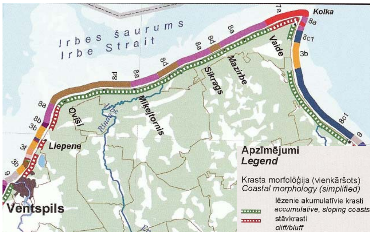
9. attēls. Baltijas jūras Kurzemes krasta ģeoloģiskā uzbūve (krasta tipi). Avots: Baltijas jūras Latvijas krasta procesi. Atlants. Guntis Eberhards, Jānis Lapinskis.
