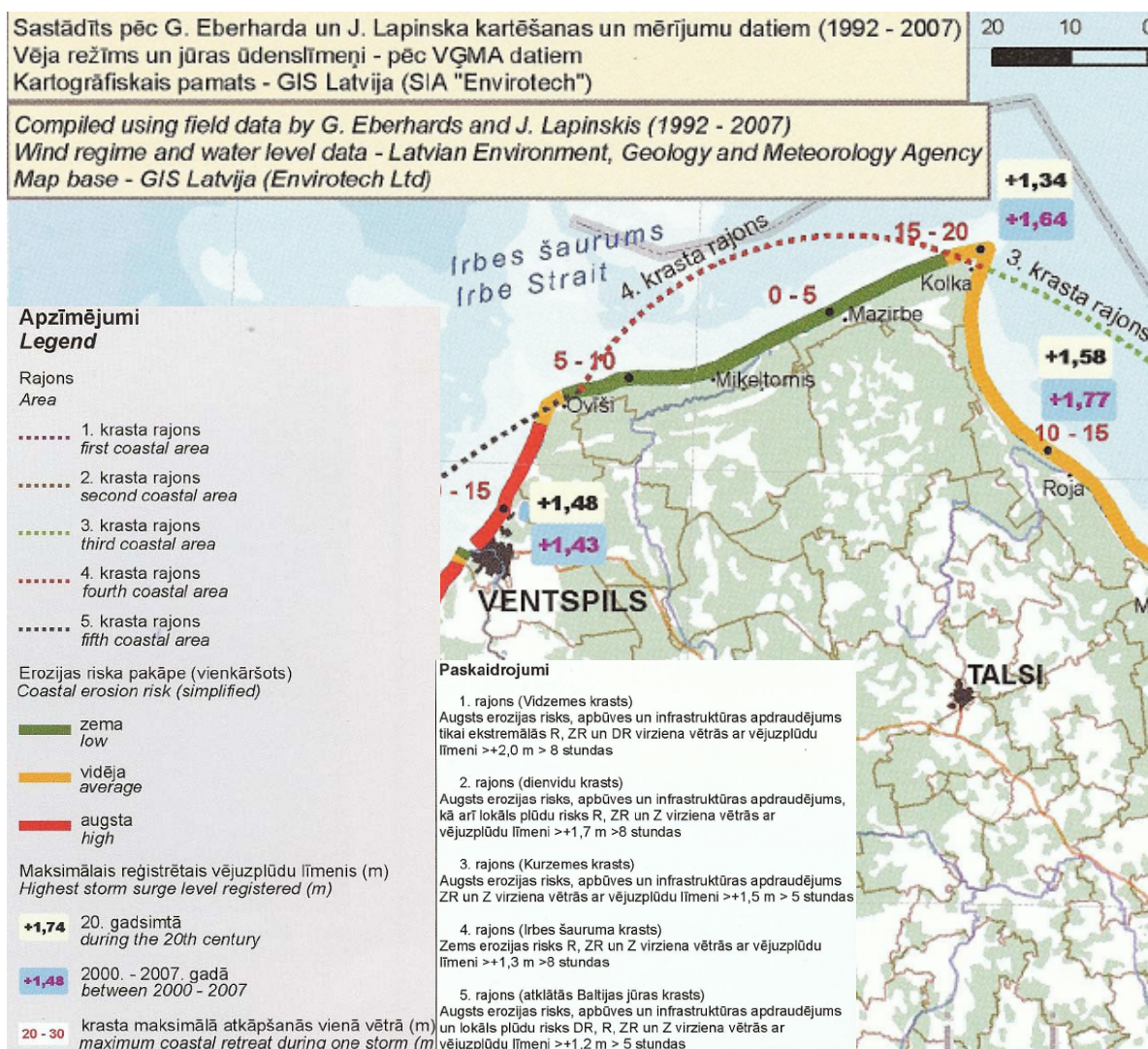
10. attēls. Latvijas jūras krasta erozijas risku noteicošie lokālie apstākļi. Avots: Baltijas jūras Latvijas krasta procesi. Atlants. Guntis Eberhards, Jānis Lapinskis.
